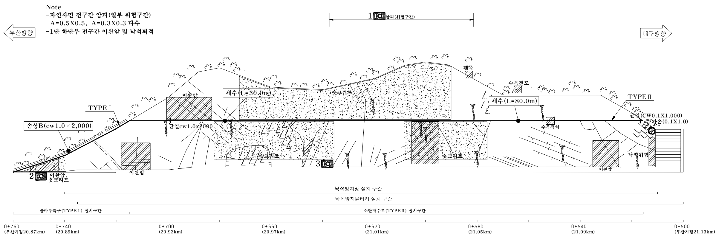
부산절토33/부산기점 20.87~21.13km (10공구 STA.0+500~0+760)
